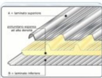
stratigrafia pannello
