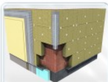
Cappotto in lana di roccia
